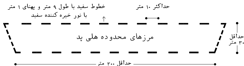
نقشه ۲-۱۶- محوطه هلی‌پد در زمین غیر مستطیلی
