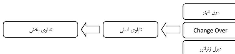
شکل ۵-۱۰-۱- بلوک دیاگرام برق‌رسانی به تابلوهای اضطراری
